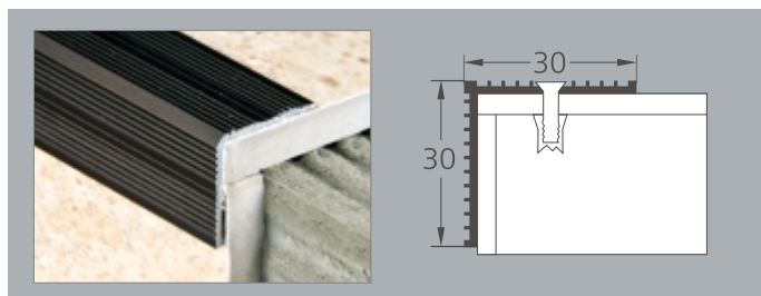
87 visible fixing color : 01, 02
