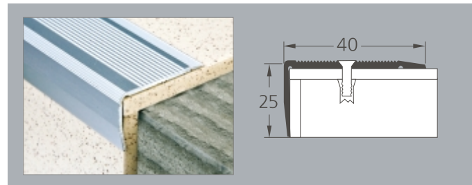
2626 invisible fixing color : 01, 02
