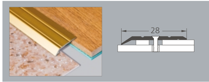
3418 visible fixing color : 01, 02
